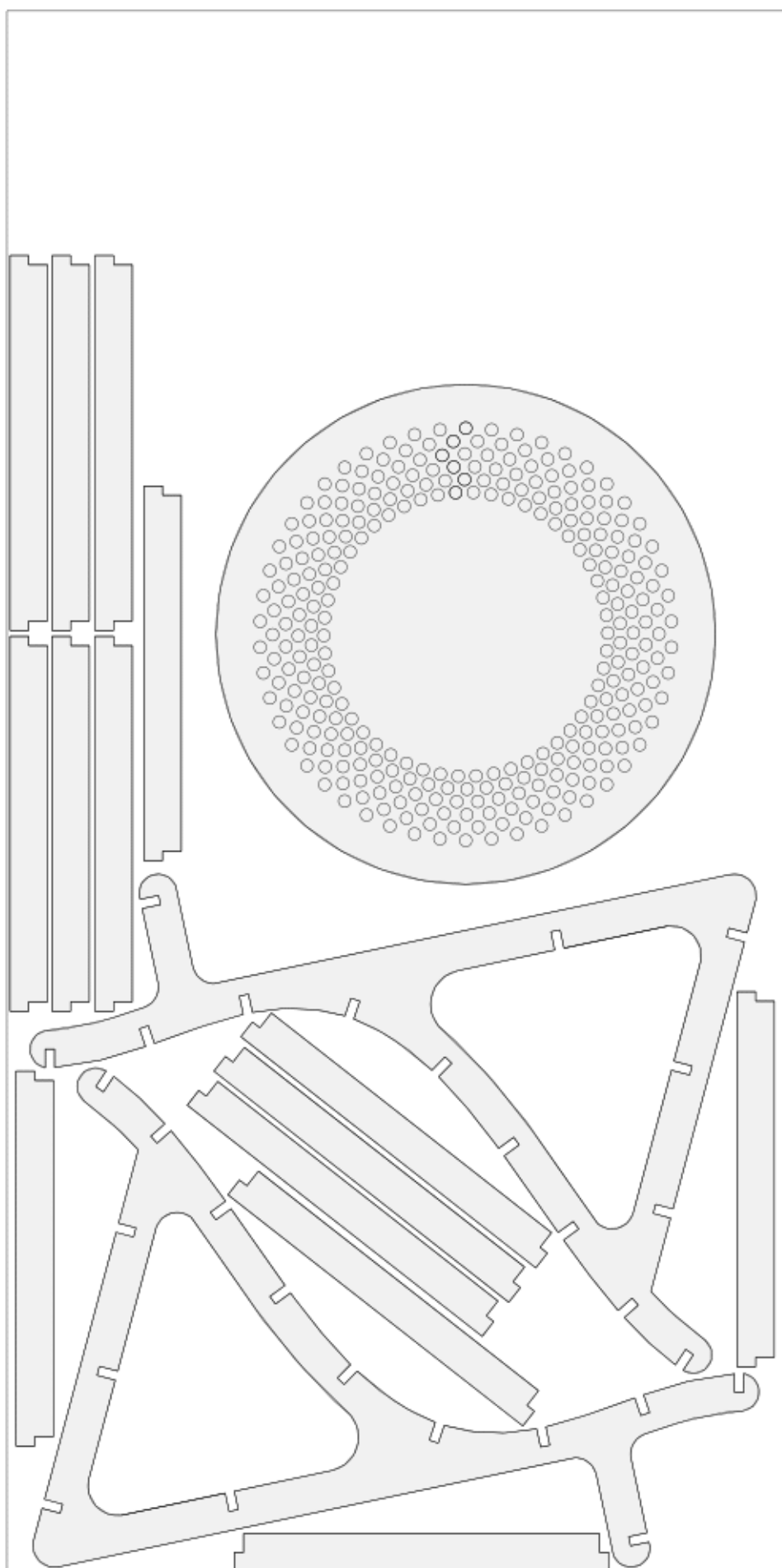
Розкрій Фанери 2500x1200x15мм
