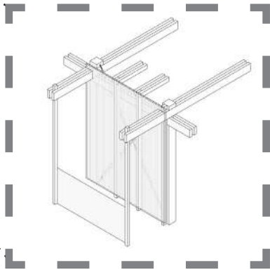
ВУЗОЛ КРИТОГО ФАСАДУ
