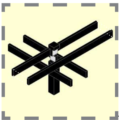
ВУЗОЛ ДЕРЕВ'ЯНОЇ КОЛОНИ
