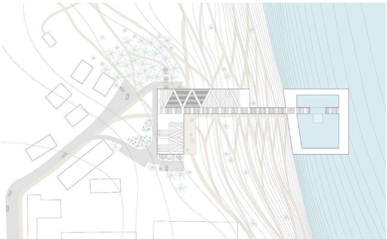
Рис 4.4 Майстерплан
